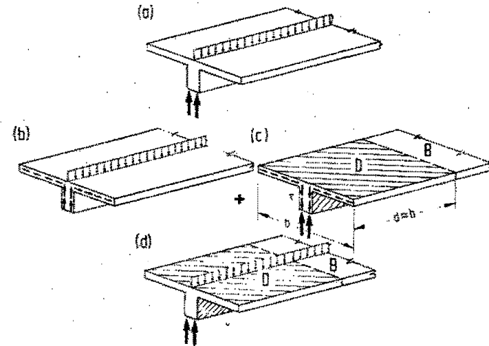
Fig. 3.4. T-beam.
